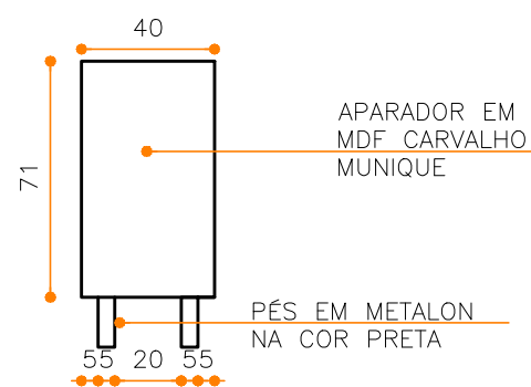
MOB.15.03- APARADOR VISTA LATERAL
