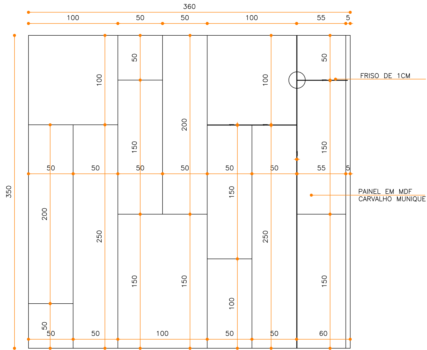
MOB.01.02 - PAINEL RECEPÇÃO VISTA 01 ESCALA 1/25
