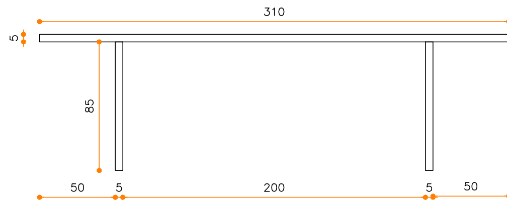
MOB.12.01 - MESA REUNIÃO VISTA FRONTAL ESCALA 1/25
