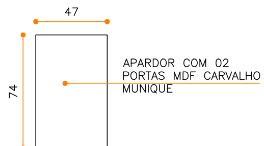
MOB.09.02 - APARADOR VISTA SUPERIOR ESCALA 1/25
