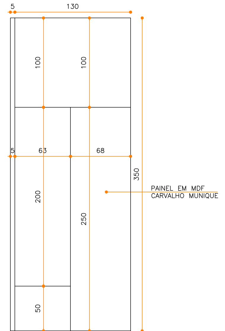
MOB.02.04 - PAINEL RECEPÇÃO 02 ESCALA 1/25
