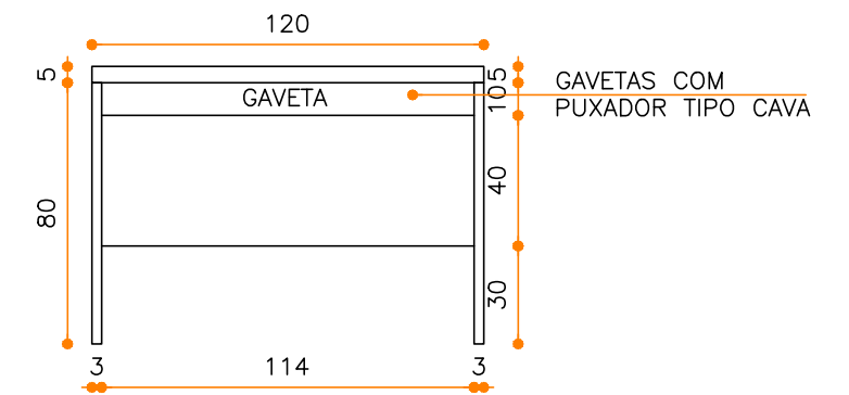
MOB.13.02 - MESA PRESIDENTE VISTA FRONTAL INTERNA ESCALA 1/25
