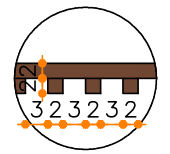
DET. 02.01 - RIPADO VISTA SUPERIOR
